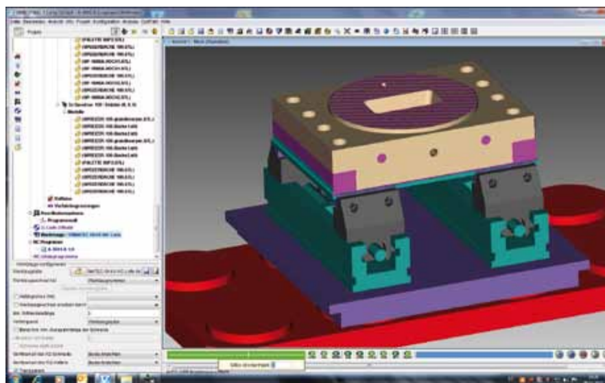
Digitale Sicherheit im digitalen Zeitalter: VERICUT® simuliert seit 2007 die CNC-Fertigung der Trimatec Mechanische Systemtechnik GmbH.
